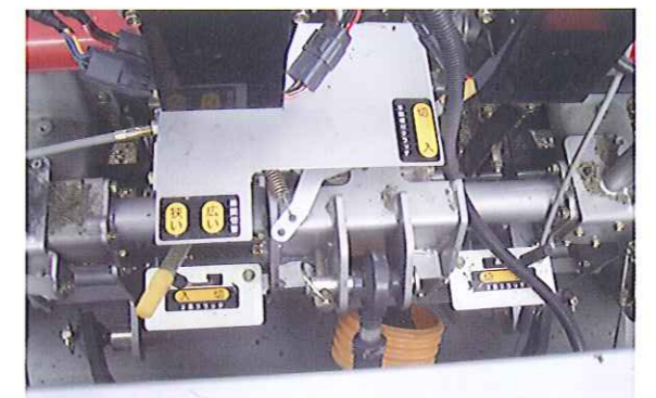
2条クラッチの採用・リフトアップ時植付けを 作動出来るクラッチレバーを採用
